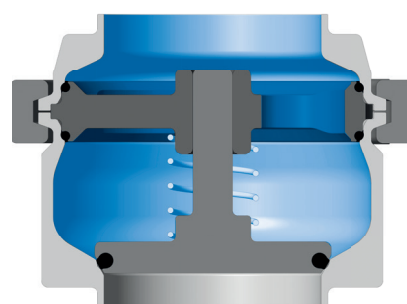
Ventilstellung: geschlossen
