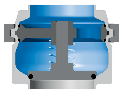
Clapet fermé
