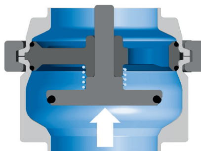
Clapet ouvert
